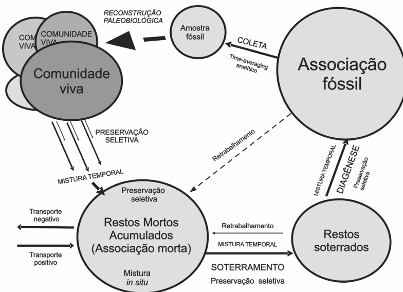
Figura 1. Diagrama mostrando as diferentes fases após a morte dos organismos até sua preservação como fósseis, e os processos que determinam vieses na análise paleobiológica final (modificado de Kidwell & Flessa 1996).
