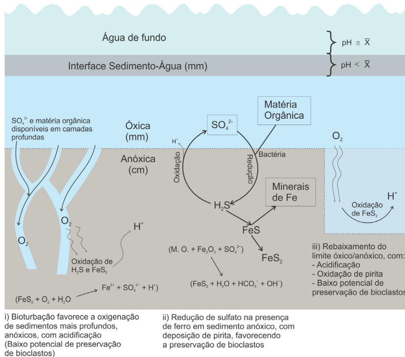
Figura 10. Série de fatores geoquímicos e diagenéticos que potencialmente podem alterar a constituição química da água de poro em sedimento marinho e, consequentemente, influenciar a taxa de destruição de conchas e esqueletos carbonáticos. Adaptado de Lovley e Phillips 1986, Lovley et al. 1993, Aller 1994, Kasten et al. 2003, Ku e Walter 2003, Haag et al. 2005.
