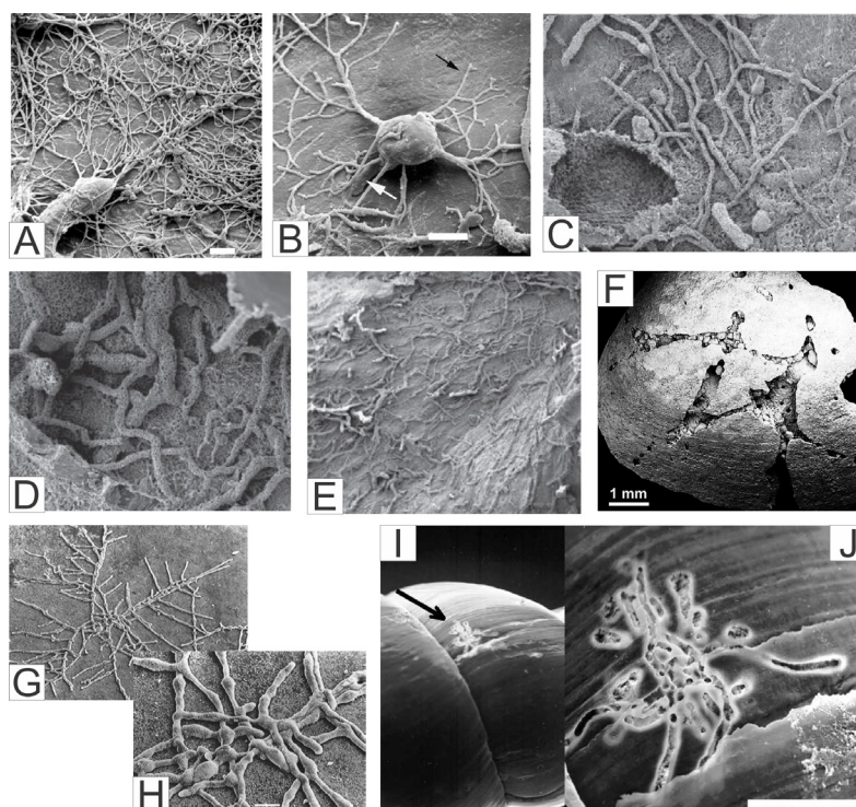
Figura 5. Exemplos de bioerosão.
