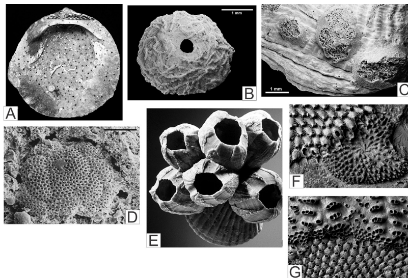
Figura 6. Exemplos de incrustação. A) Interior de um bivalve ( Glycymeris ) incrustado por serpulídeos, briozoários, e bioerodido por esponja ( Cliona sp.). Foraminíferos: B) Rosalina spp. C) Cornuspiramia antillarum . D) Homotrema rubrum . E) Cracas ( Megabalanus sp.) incrustadas em uma concha de bivalve. Incrustação por briozoários: F) Escharoides sp. sobrecrecendo Liripora sp. (aumento de 13x), G) Desmediaperocia sp. sobrecrecendo briozoário quilóstomo (aumento de 18x). Adaptado de Taylor e Wilson (2002; 2003) e Hauser et al. 2008.
