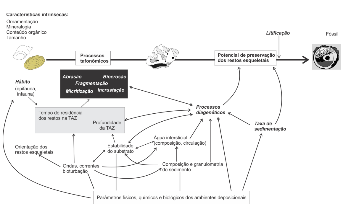
Figura 2. Aspectos que influenciam a alteração dos restos bioclásticos após a morte até a fossilização (adaptado de Stienne, 2010).
