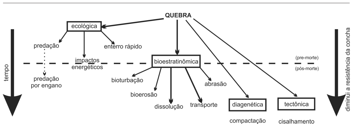
Figura 7. Esquema generalizado dos fatores que influenciam a fragmentação de conchas em meio marinho (modificado de Zuschin et al. 2003).
